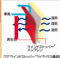
ゴア®ウインドストッパー®ファブリクス構造図
